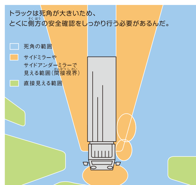
■トラックの死角と歩行者などとの関係
