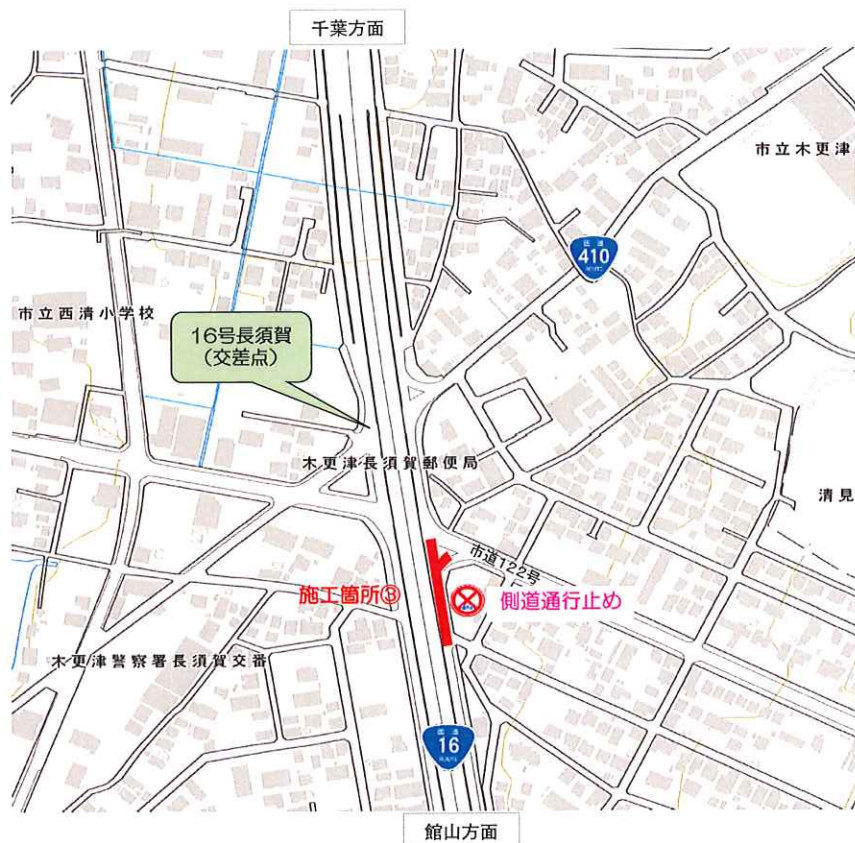
工事施工箇所位置図
